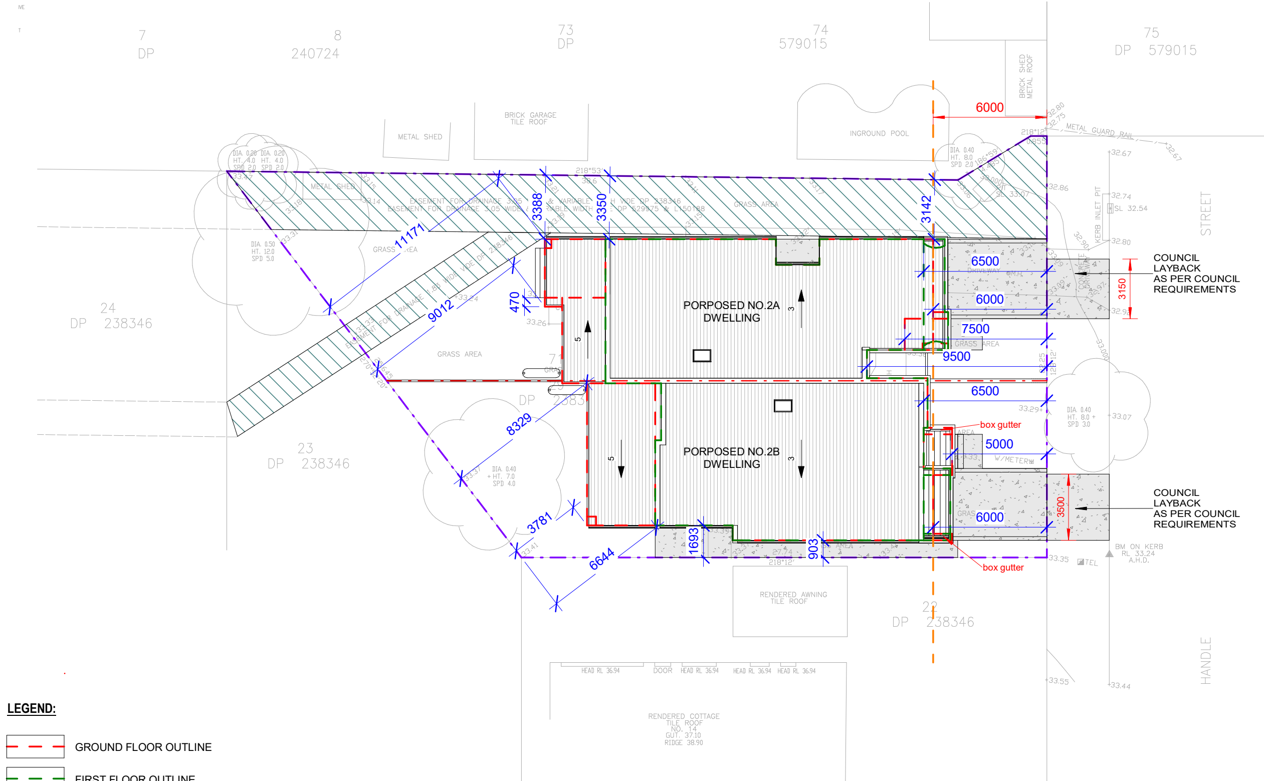
1 SITE PLAN & ROOF PLAN, SITE ANALYSIS PLAN 1 : 200
